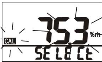
Afb. 28: Kalibrering van de luchtvochtigheidssensor
