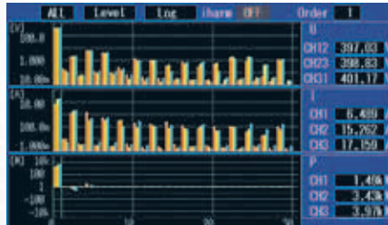
RMS values
